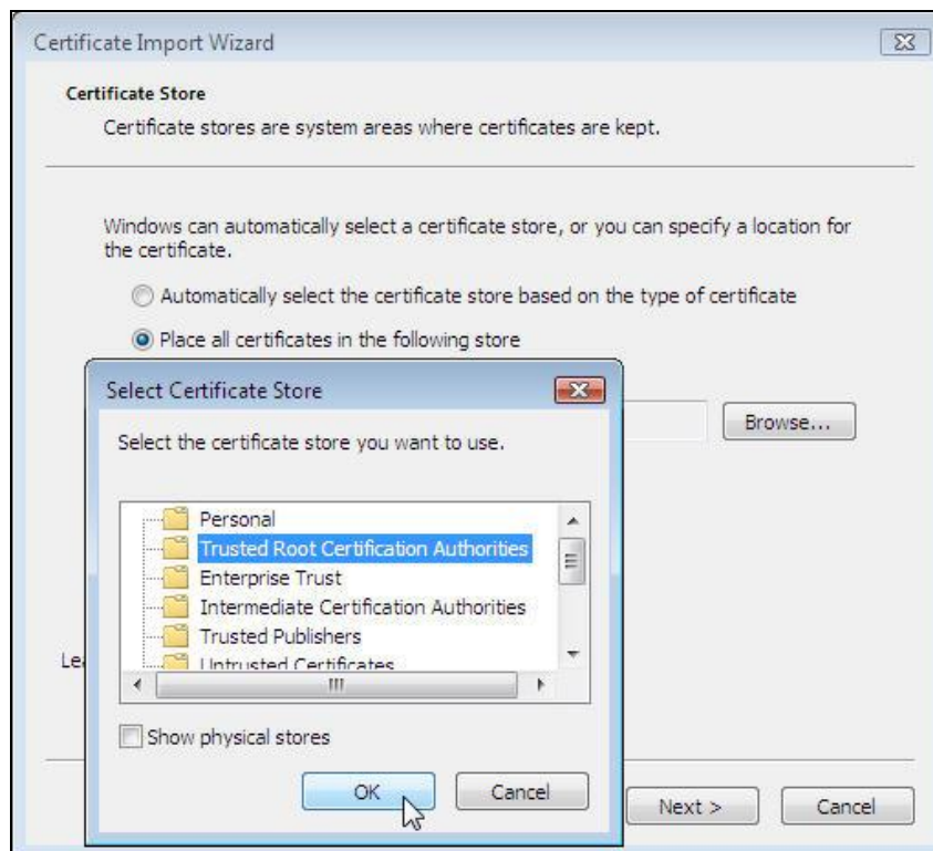
Slika 6. Forma za izbor skladišta sertifikata Internet Explorer-a (Windows Vista)
